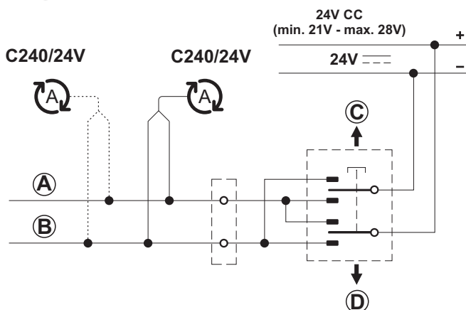
Fig. 44 C240/24V
